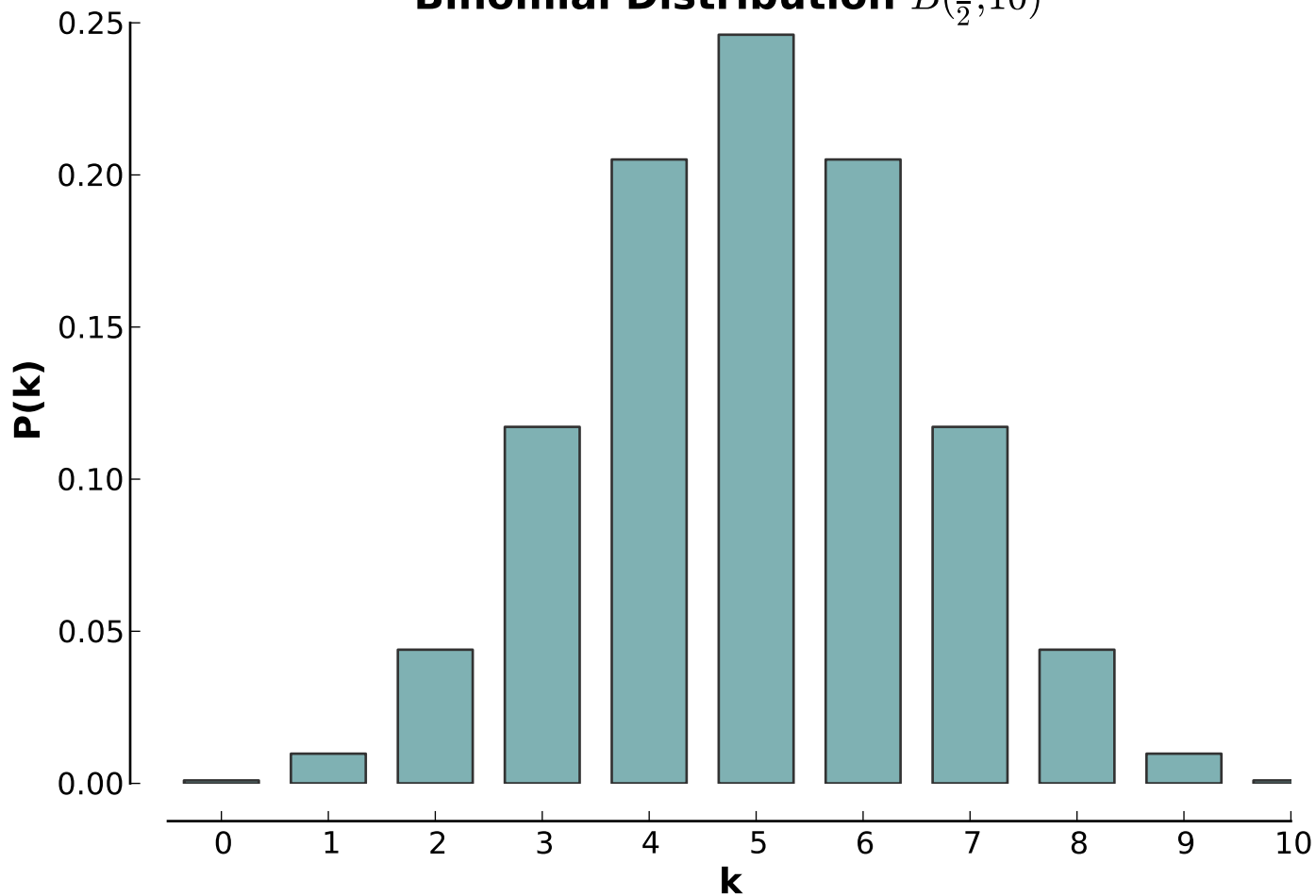
Binomial Distribution B(\frac{1}{2}, 10)
