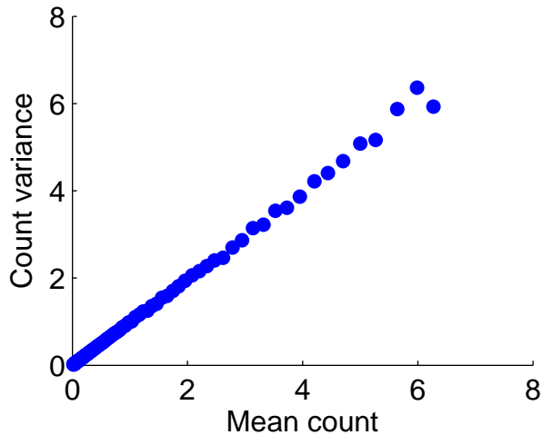
Poisson
