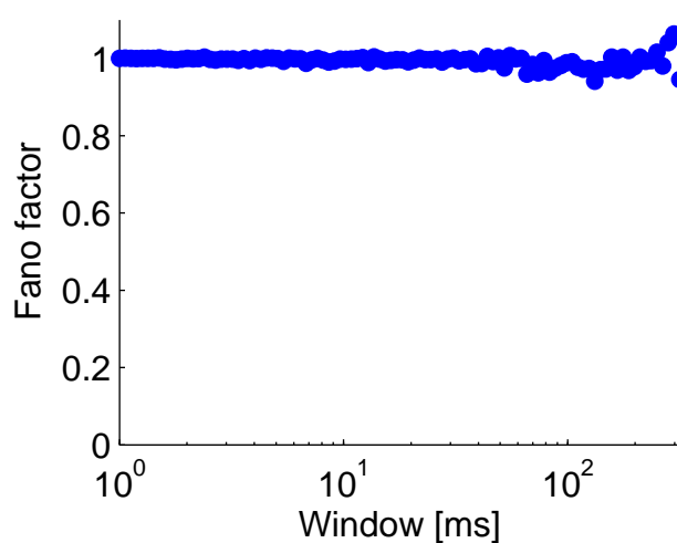
Poisson
