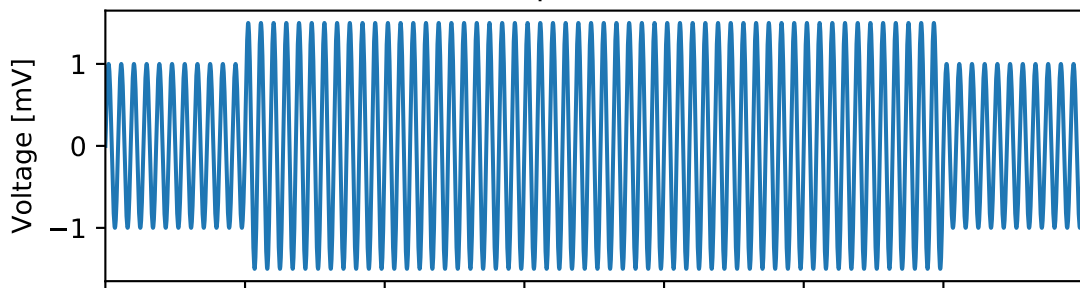
SAM Stimulus
